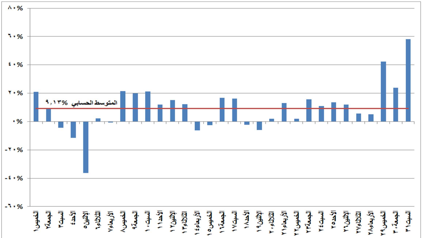
شكل (٢٢) نسب التغير في استخدام المصادر غير الحرارية في إنتاج الطاقة الكهربائية خلال شهر مارس ٢٠١٨ مقارنة بالشهر المماثل من العام السابق
