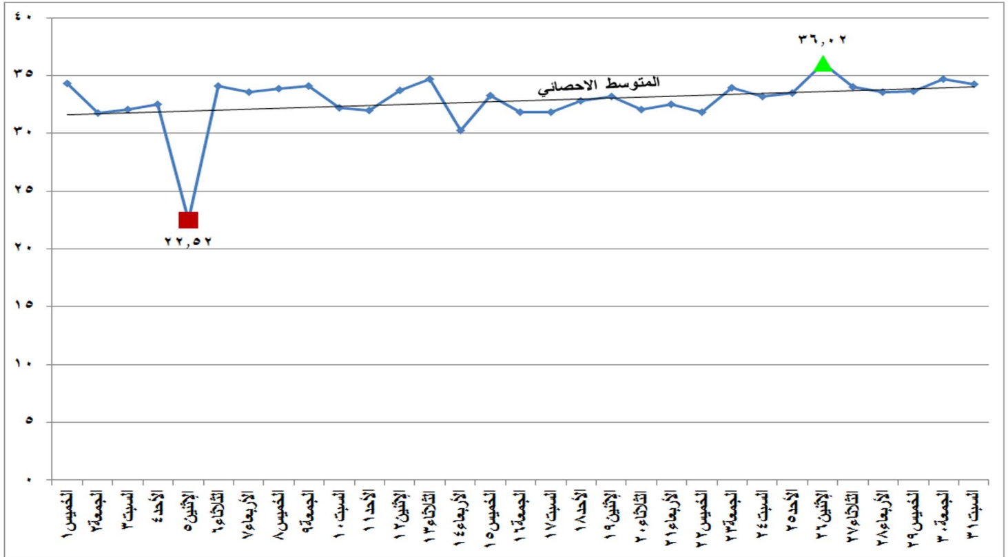
شكل (٢٣) الطاقة الكهربائية المنتجة من المصادر المائية خلال شهر مارس ٢٠١٨
