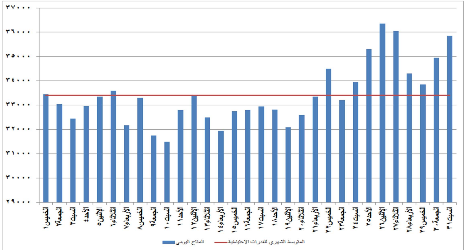
شكل (٢٧) القدرات المتاحة يوميا والمتوسط الشهري للقدرة الاحتياطية خلال شهر مارس ٢٠١٨
