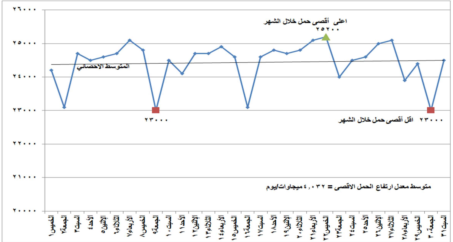
شكل (١) تطور الحمل الاقصى اليومي خلال شهر مارس ٢٠١٨
