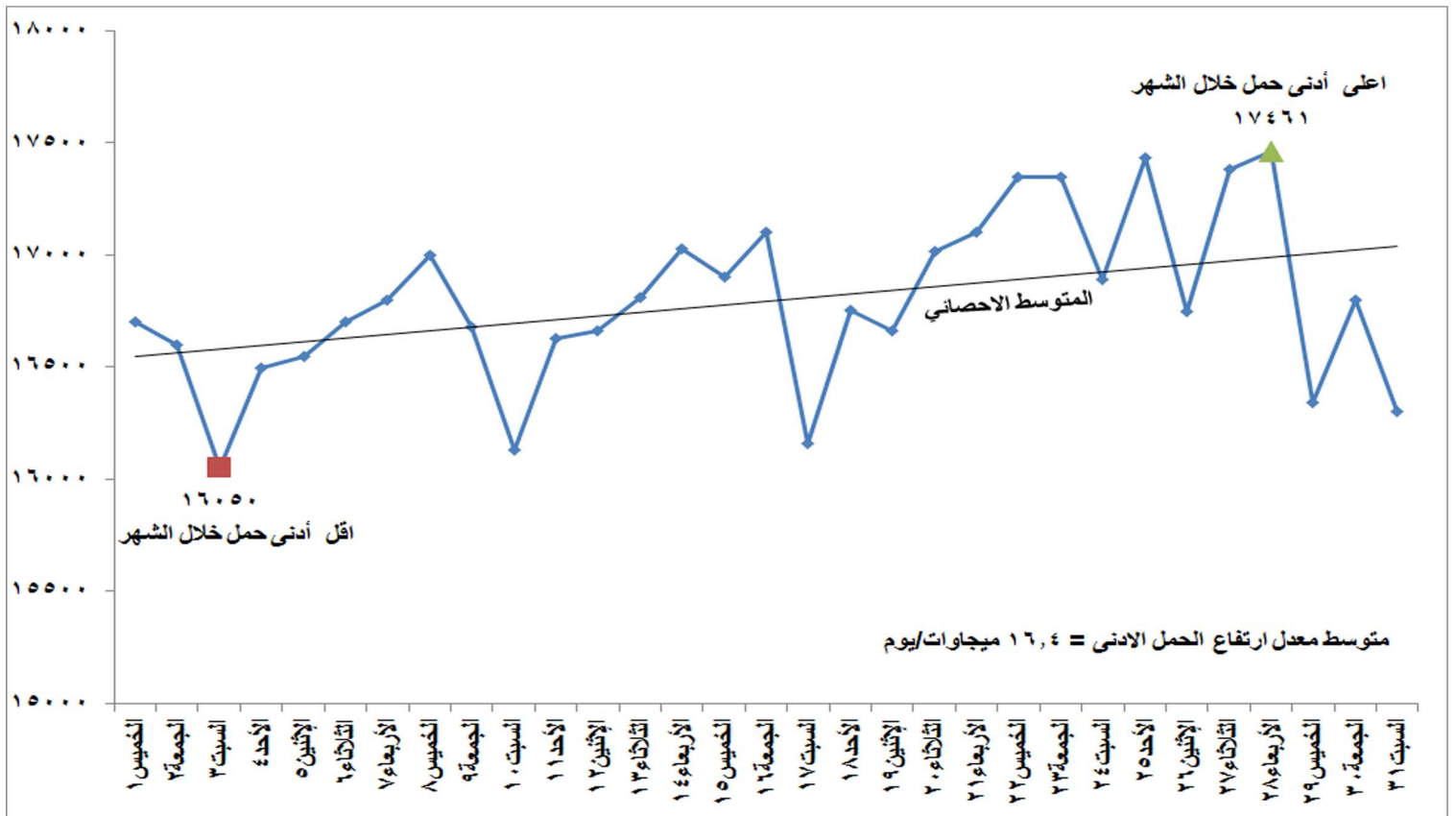
شكل (٢) تطور الحمل الادنى اليومي خلال شهر مارس ٢٠١٨
