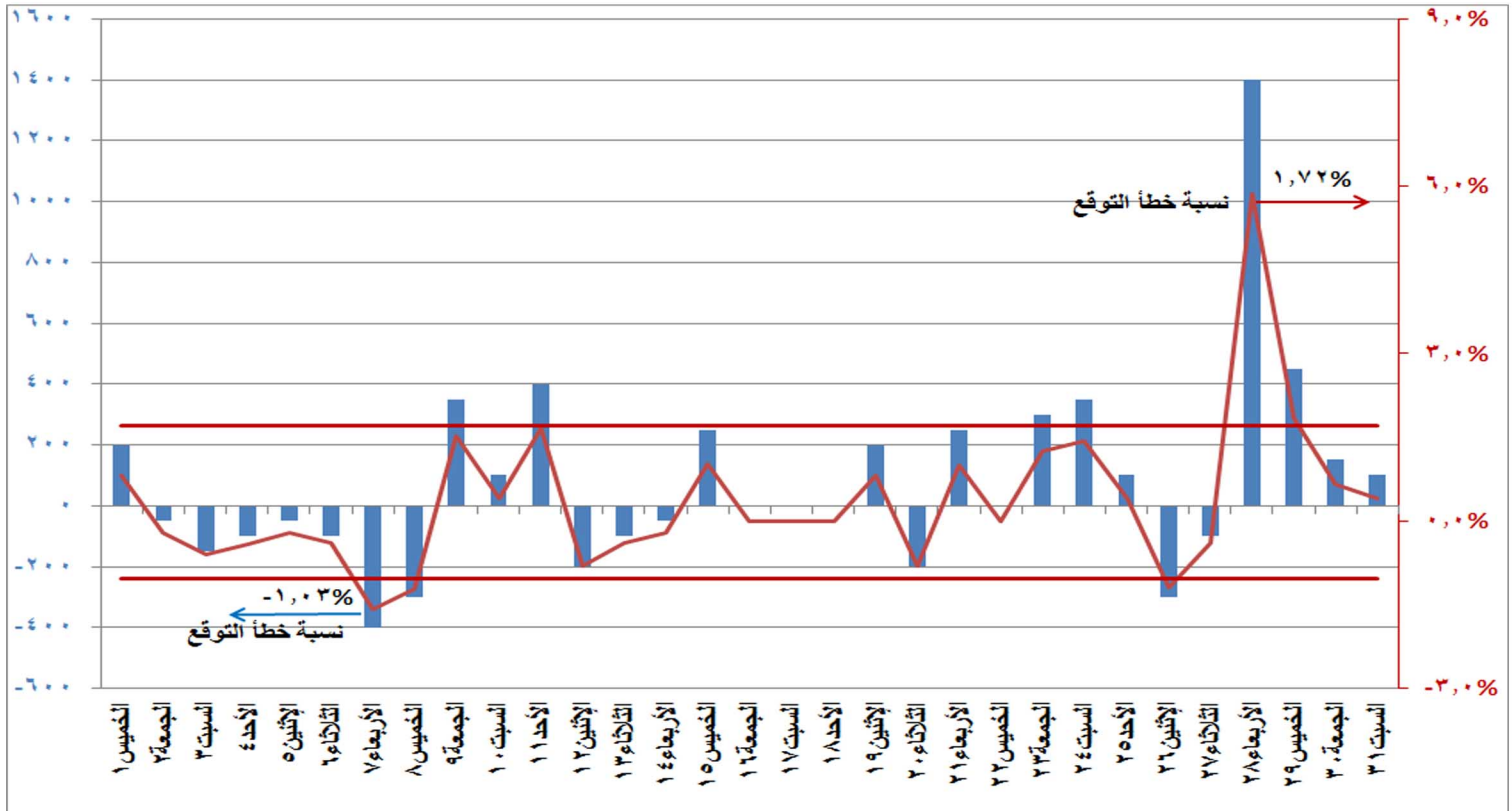
شكل (١٠) الفرق بين الحمل الأقصى المتوقع والمسجل فعليا ونسبة الفرق إلى الحمل المسجل فعليا خلال شهر مارس ٢٠١٨
