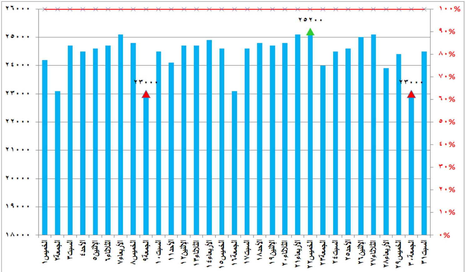
شكل (٥) قدرات الانتاج المتاحة ونسبتها للحمل الأقصى خلال شهر مارس ٢٠١٨
