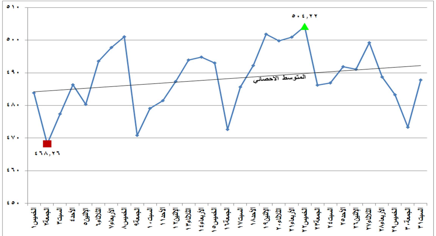
شكل (١٥) إجمالي الطاقة الكهربائية المنتجة من كل المصادر الأولية خلال شهر مارس ٢٠١٨
