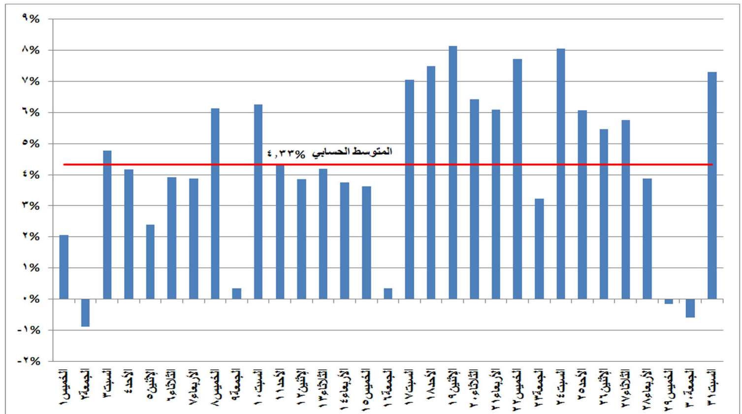
شكل (١٦) نسب التغير في الطاقة الكهربائية المنتجة خلال شهر مارس ٢٠١٨ مقارنة بالشهر المماثل من العام السابق
