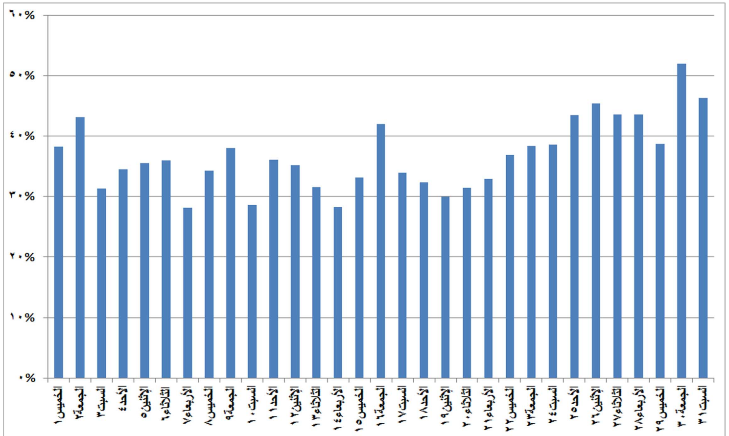
شكل (٢٨) نسب الفائض للحمل الاقصى المسجل يوميا خلال شهر مارس ٢٠١٨
