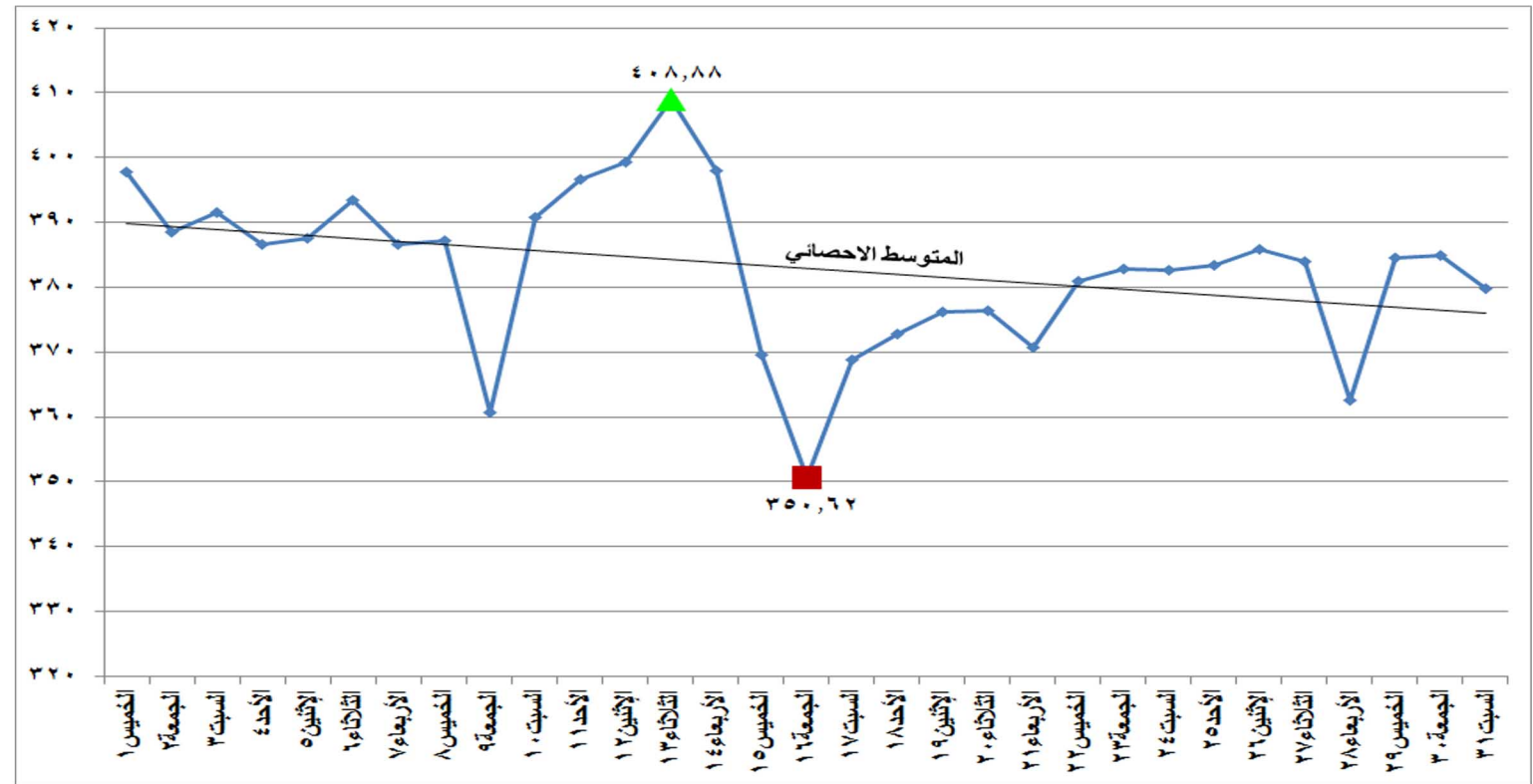
شكل (١٧) الطاقة الكهربائية المنتجة من الغاز الطبيعي خلال شهر مارس ٢٠١٨
