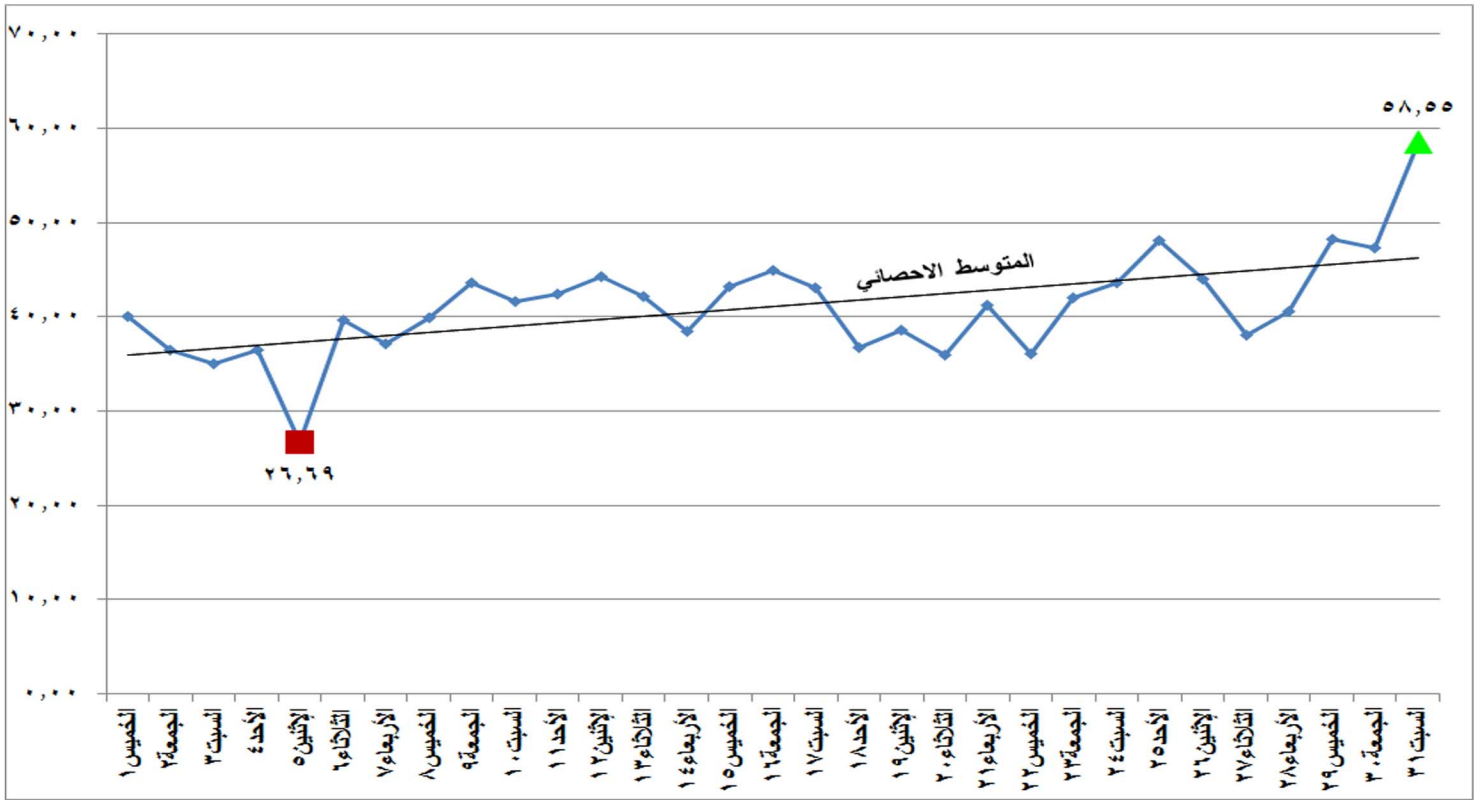
شكل (٢١) الطاقة الكهربائية المنتجة من المصادر غير الحرارية خلال شهر مارس ٢٠١٨
