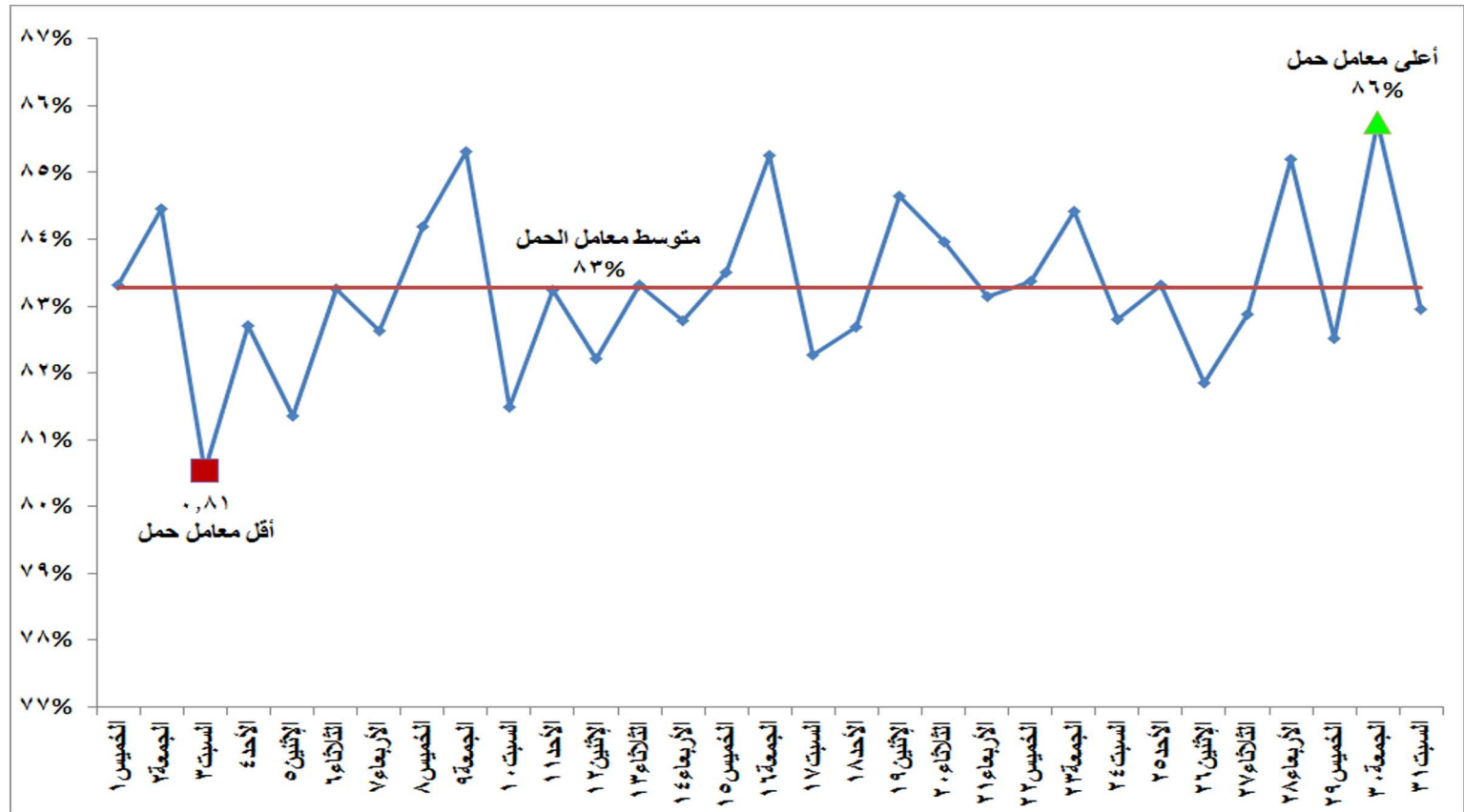
شكل (١٢) إجمالي معامل الحمل لوحدات الانتاج خلال شهر مارس ٢٠١٨
