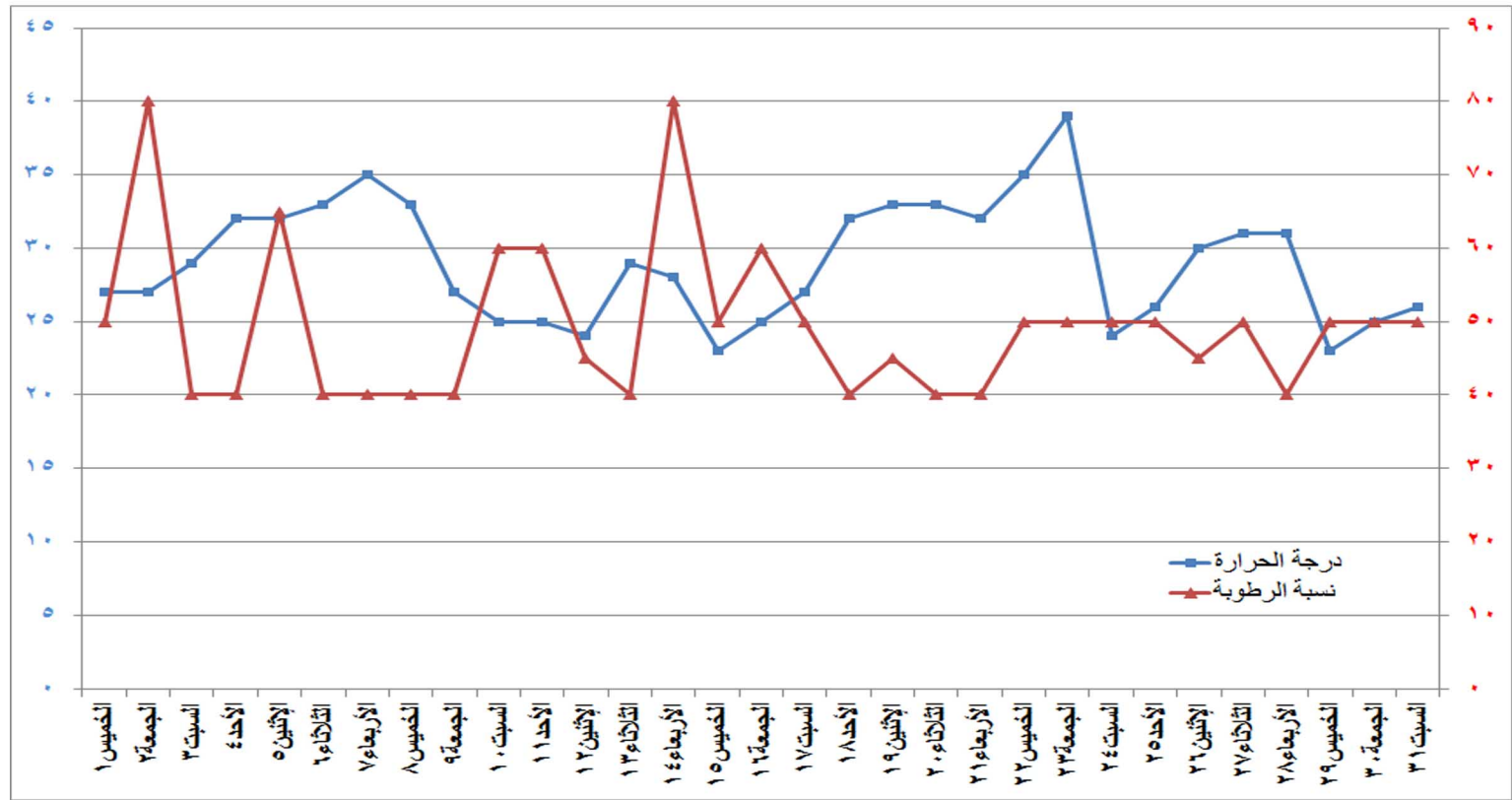
شكل (١١) التغيير في درجة الحرارة والرطوبة النسبية خلال شهر مارس ٢٠١٨
