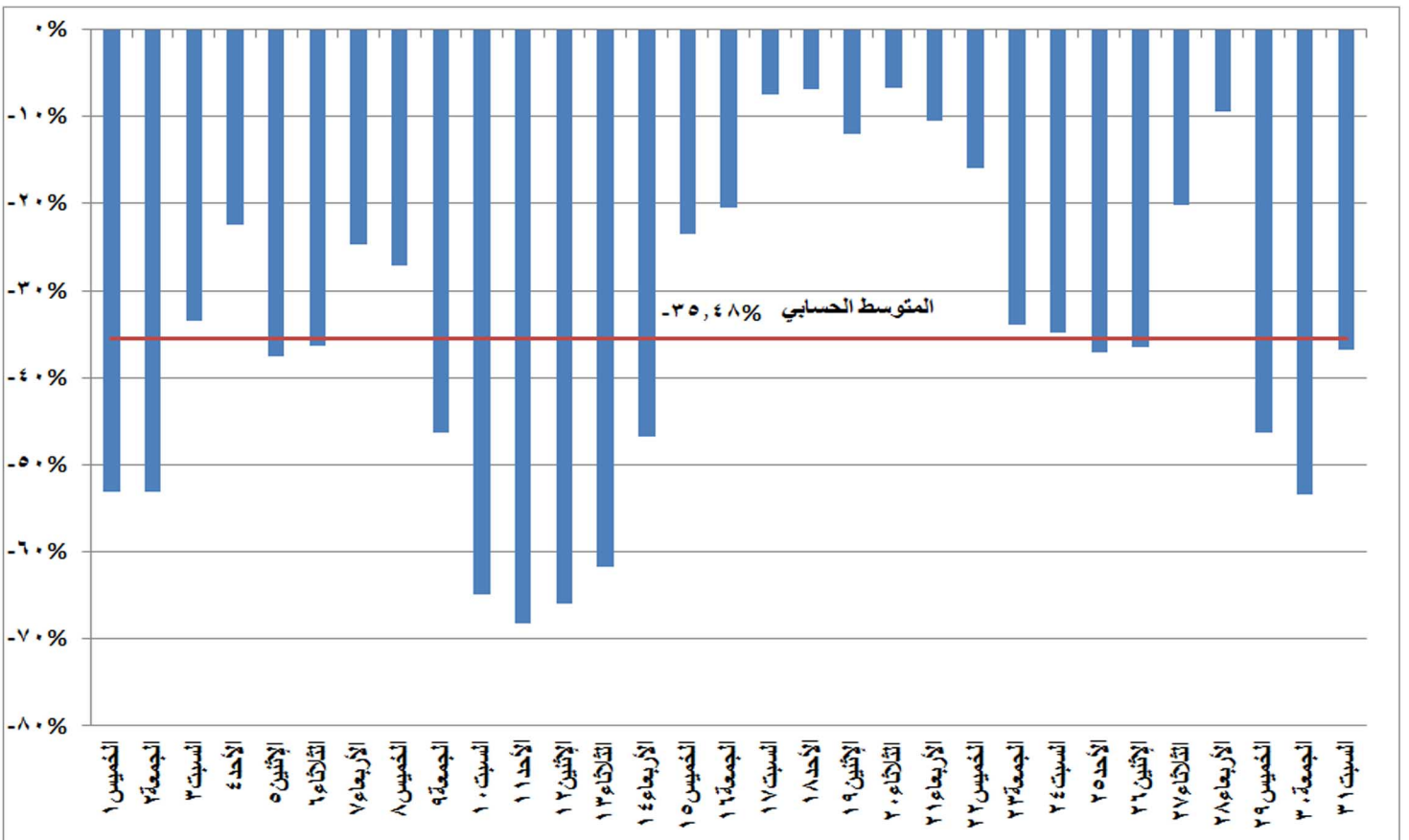
شكل (٢٠) نسب التغير في استخدام المازوت في إنتاج الطاقة الكهربائية خلال شهر مارس ٢٠١٨ مقارنة بالشهر المماثل من العام السابق
